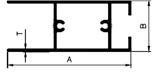
TOP BOTTOM
