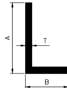
UNEQUAL ANGLE
